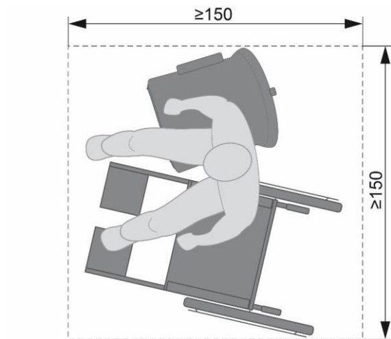
Abb. 1: Mindestgröße der Bewegungsfläche für das Umsetzen (Maße in cm)
